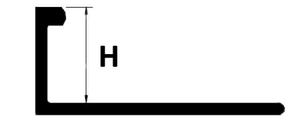
YJ-SE H:6/8/10/12mm
